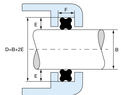
Stangafdichting
