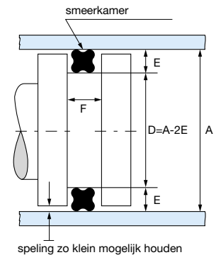
Zuigerafdichting
